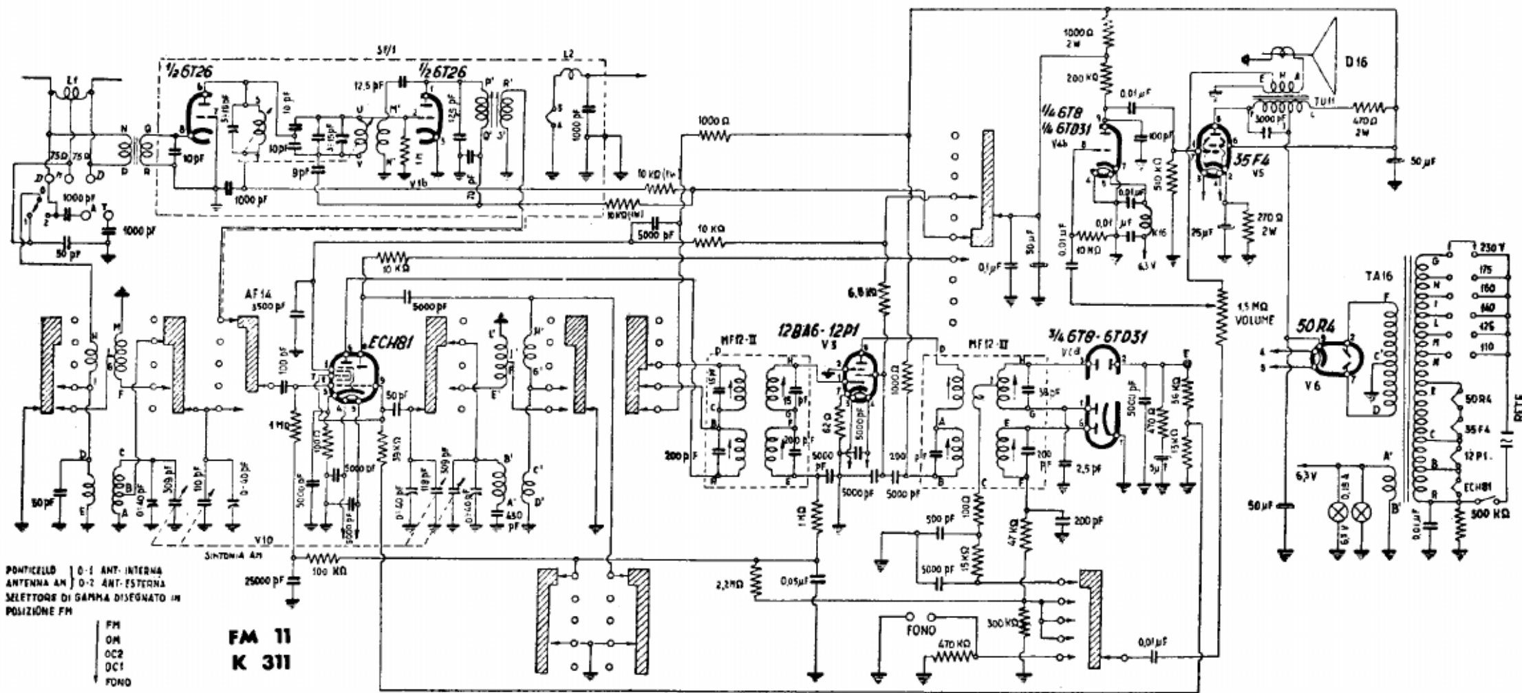
MAGNADYNE RADIO - Mod. FM 11 e K 311. Apparecchio a modulazione d'ampiezza e di frequenza. Onde medie, due gamme onde corte e una banda onde ultracorte a modulazione di frequenza. Media frequenza AM a 471 kc/s, e FM a 10,7 Mc/s. Potenza d'uscita 4 watt.
